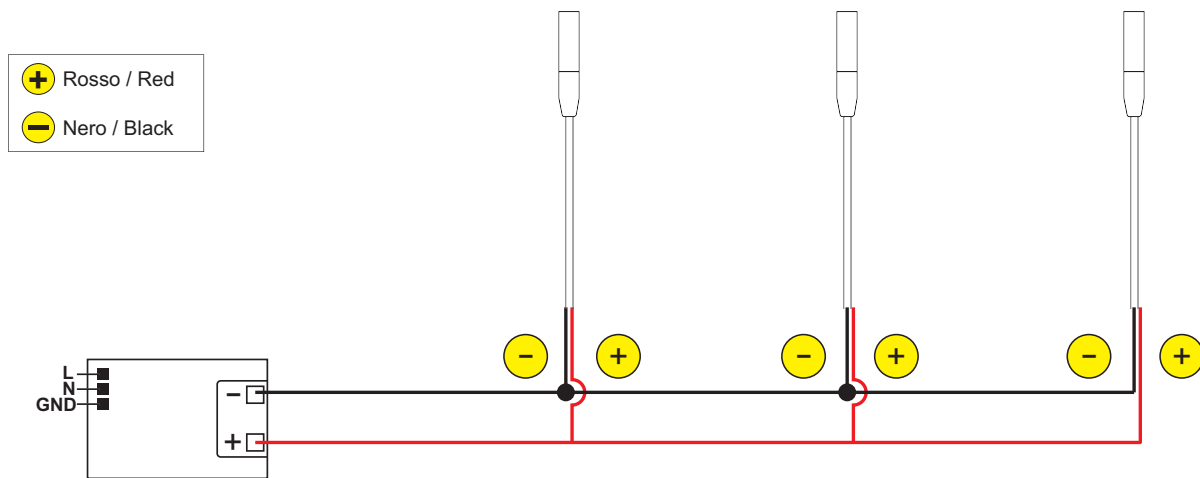
Schema di connessione in parallelo per versione 24V - Connection diagram for 24V version
