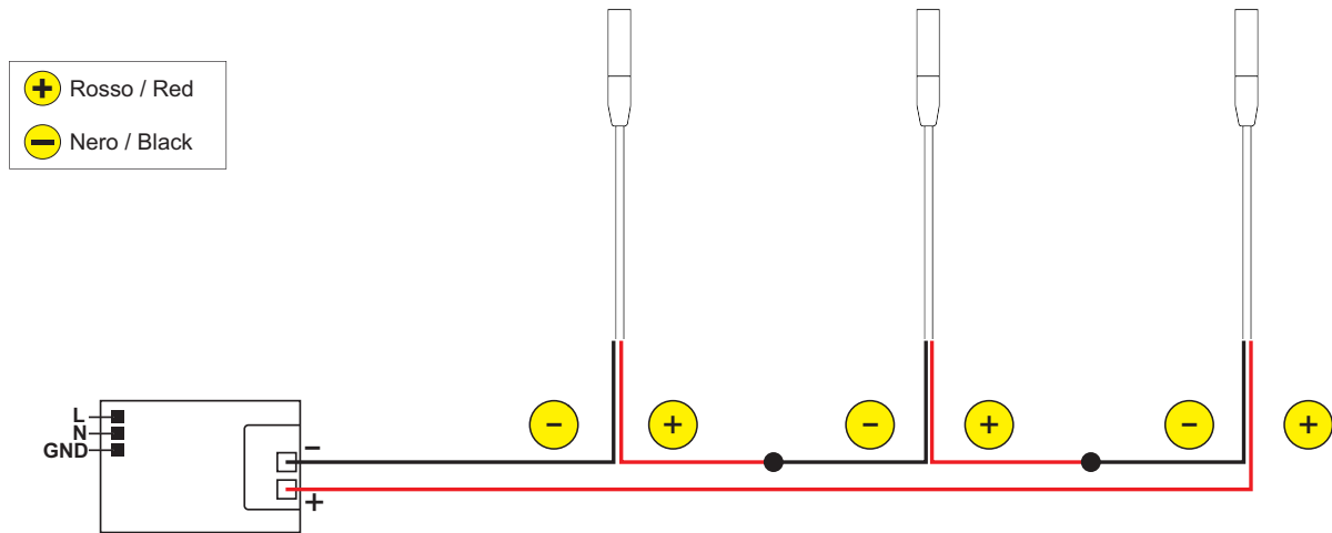
Schema di connessione in serie per versione 350 / 500 / 700mA - Connection diagram for 350 / 500 / 700mA version
