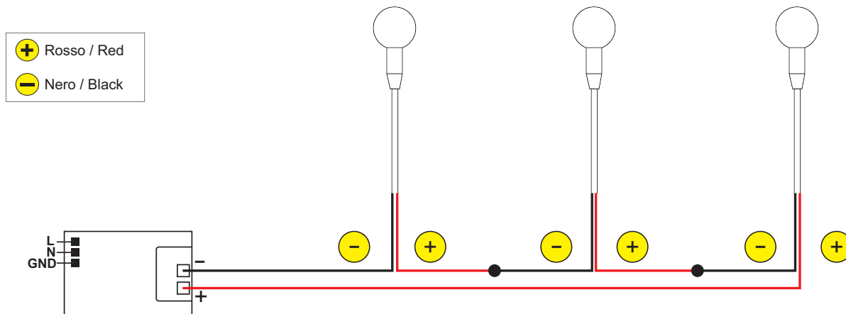
Schema di connessione in serie per versione 350 / 500 / 700mA - Connection diagram for 350 / 500 / 700mA version
