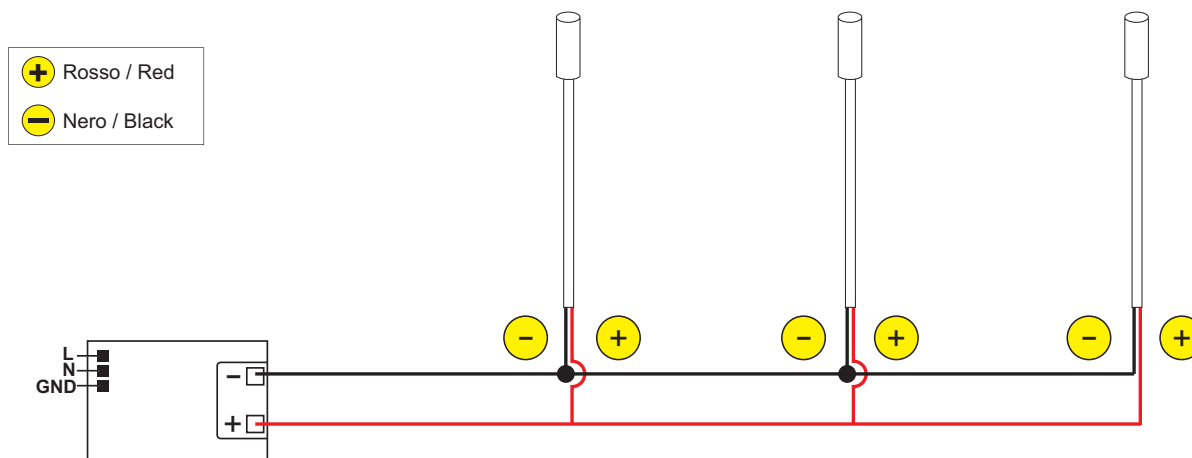
Schema di connessione in parallelo per versione 24V - Connection diagram for 24V version
