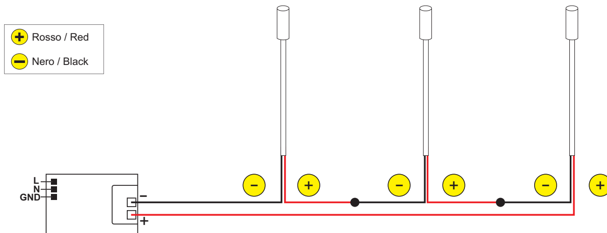
Schema di connessione in serie per versione 350 / 500mA - Connection diagram for 350 / 500mA version
