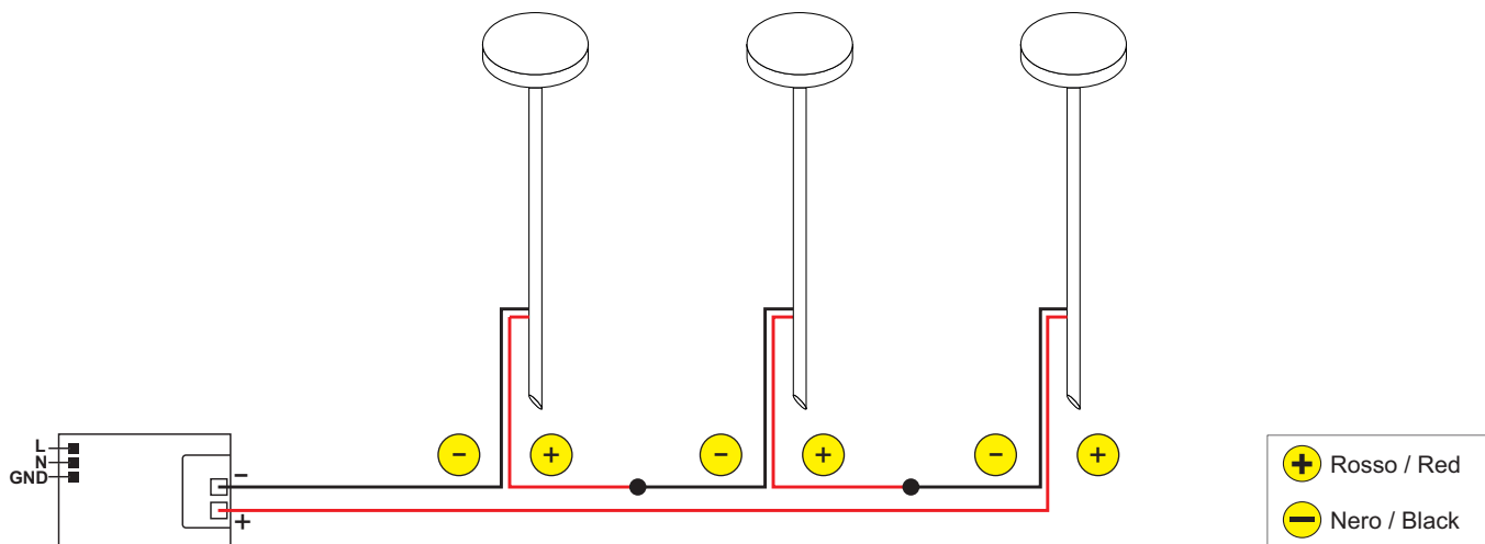
Schema di connessione in serie per versione 350 / 500mA - Connection diagram for 350 / 500mA version
