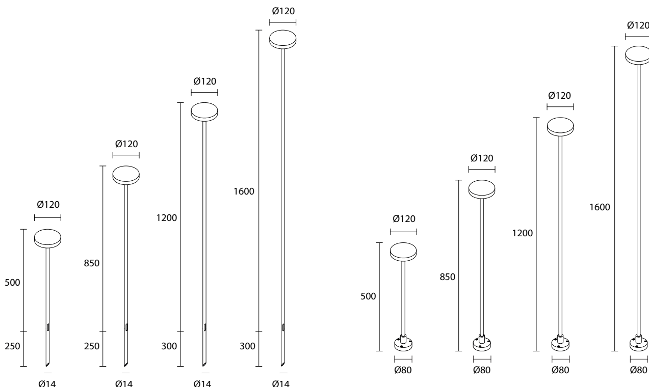
Con picchetto / With stake ( SPL01 )
