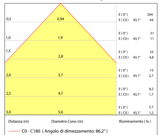
JH001: Emissione luminosa / Diagramma conico
